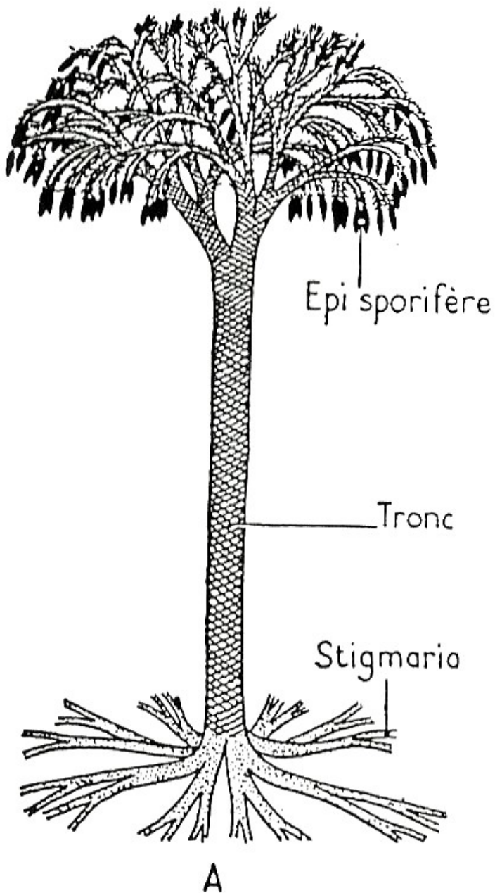
A : morphologie du lépidodendron. (Lycophyte 1 )
